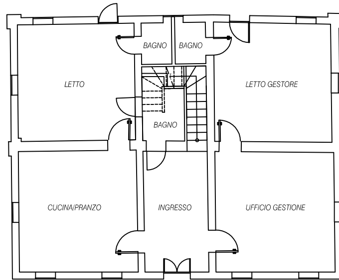
PIANTA PIANO TERRA H= 293 CM.
