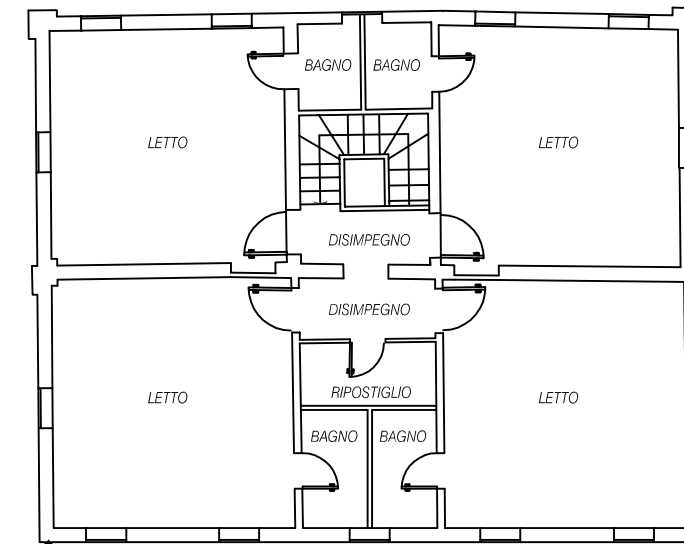
PIANTA PIANO PRIMO H= 300 CM.
